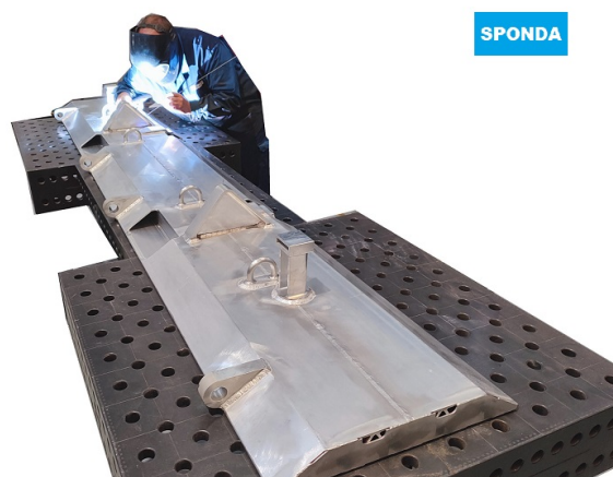
Dettaglio operazione di saldatura
